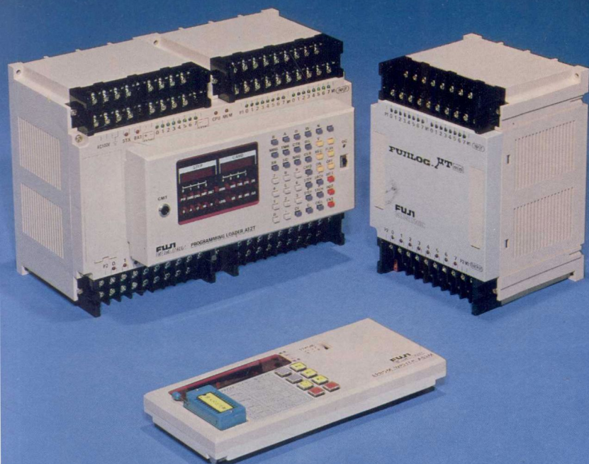
可编程序控制器 FUJI LOG系列
