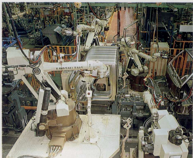
工业用自动控制装置机器人
