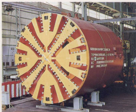
盾构挖土机
