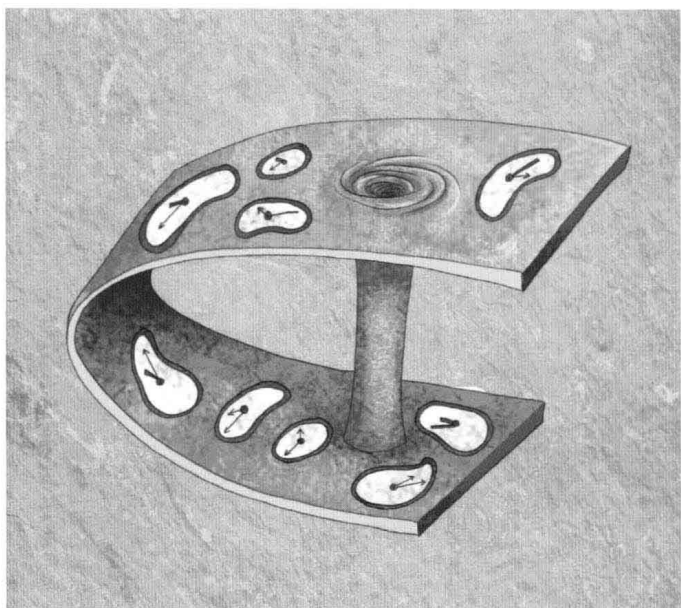
彩插5 虫洞 / P146
