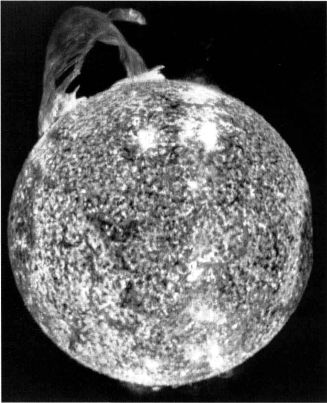
彩插3 太阳黑子 / P64
