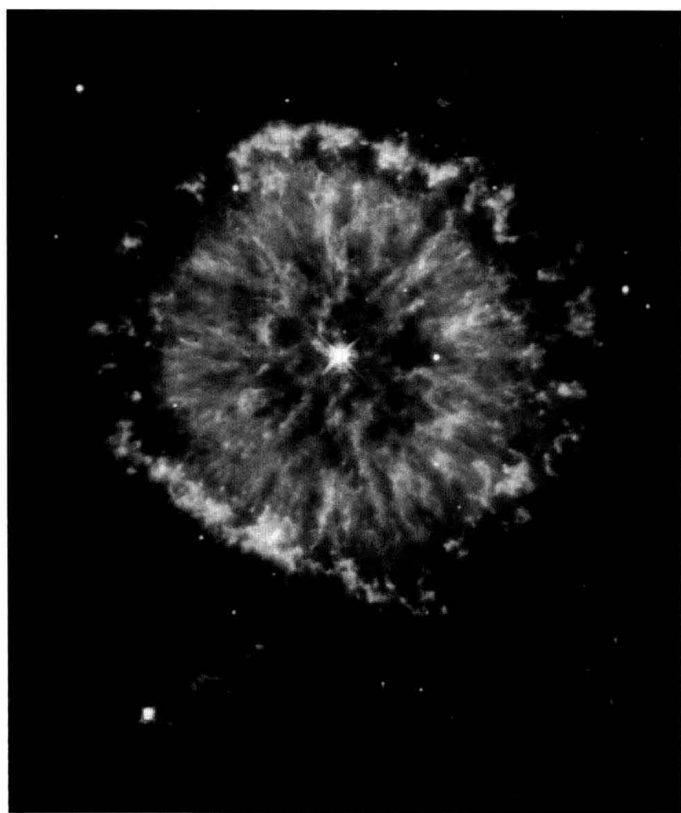
彩插6 哈勃望远镜拍摄的星云图 / P217
