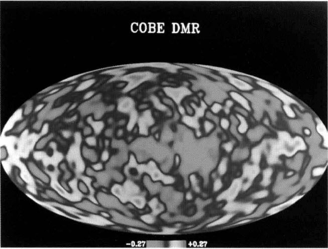
彩插2 宇宙微波背景辐射图 / P63
