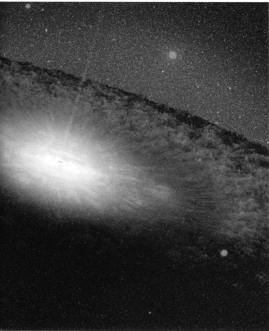
彩插4 宇宙某星系中的大黑洞 / P138
