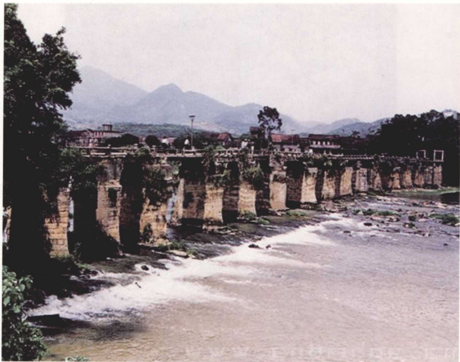
石马桥——福建仙游
