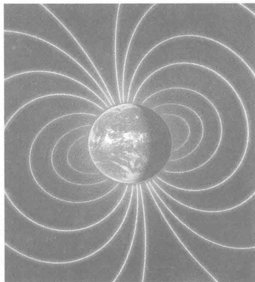
地球磁场
