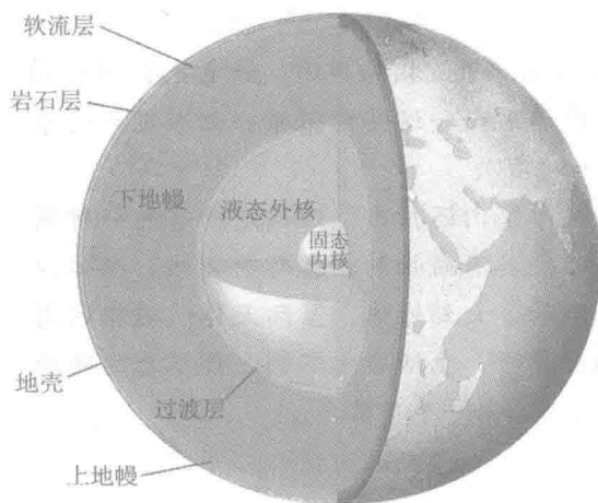
地球内部结构示意图
