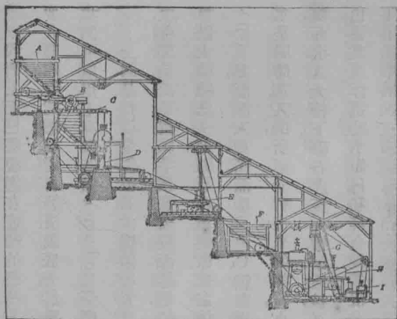
第六圖 連續方法的搗礦機底橫斷圖
