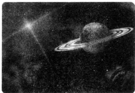
宇宙的起源问题，仍然值得人类探究
