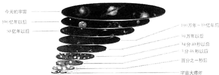
宇宙成长示意图
