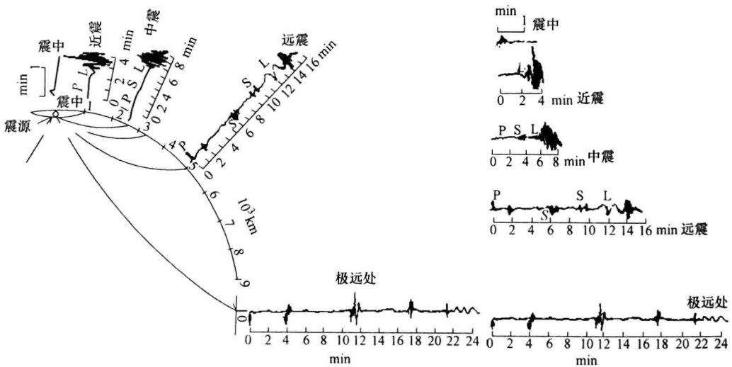
图 1.1.7 不同震中距的地震波
