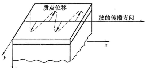
图 1.1.5 勒夫波
