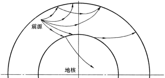
图 1.1.6 体波传播途径示意图
