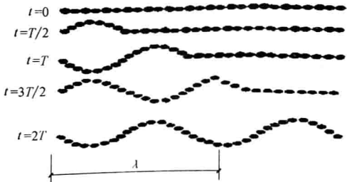
图 1.1.3 横波（S 波）
