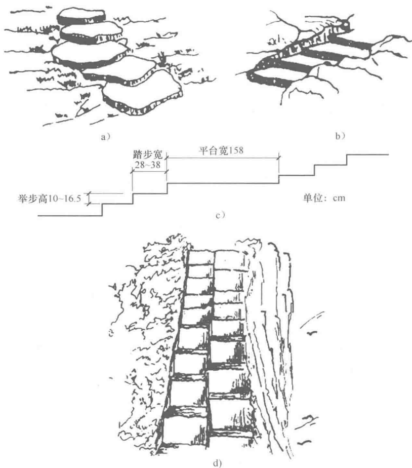
图 1-4 台阶与蹬道
