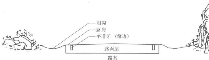
图 1-2 路堤型
