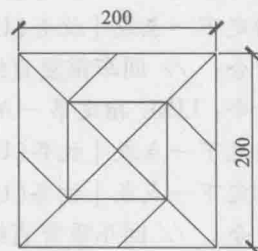
图 1-5 捕捉实例(一)
