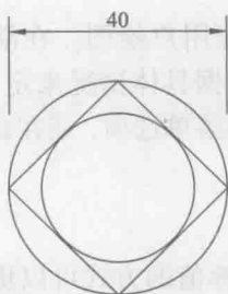
图 1-7 捕捉实例(二)
