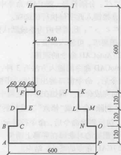
图 1-4 正交实例
