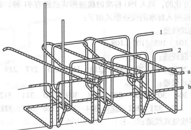
图 1-16 多根缝线互连的线迹
