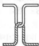
图 1-5 一根缝线与另一根缝线的交织
