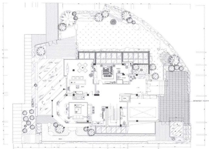
一层平面图
