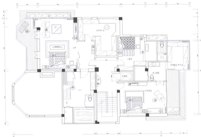
二层平面图
