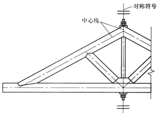
图1-8 对称符号
