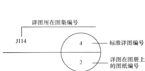
图 1-19 标准图索引
