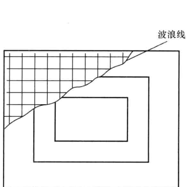
图 1-12 波浪线
