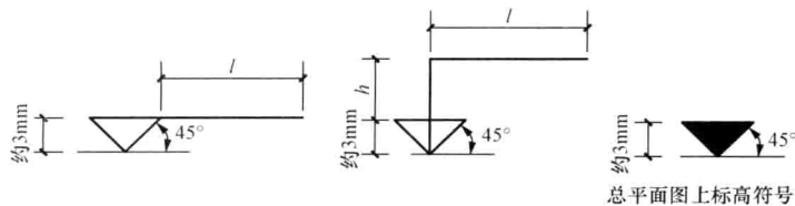
图 1-13 标高绘法
