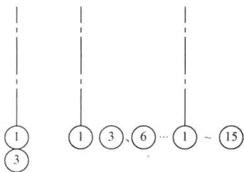
图 1-2 轴线标法
