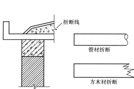
图 1-10 折断线表示方法
