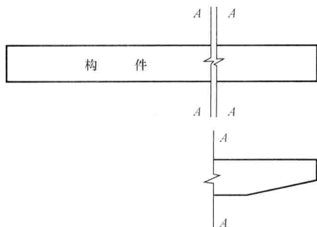
图 1-22 连接符号
