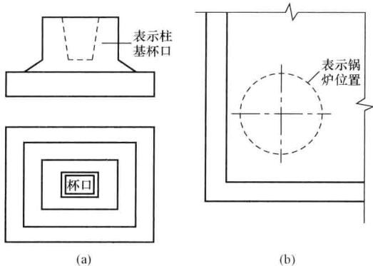
图 1-11 虚线
