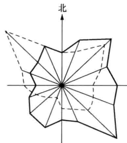
图 1-16 风玫瑰
