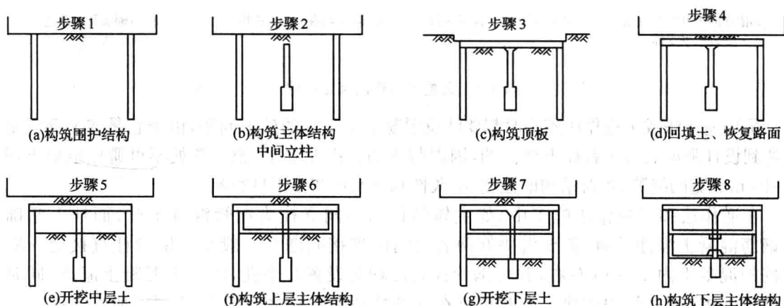
图 1.3 盖挖逆作法的一般步骤
