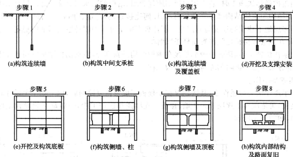
图 1.2 盖挖顺作法的一般步骤示意图
