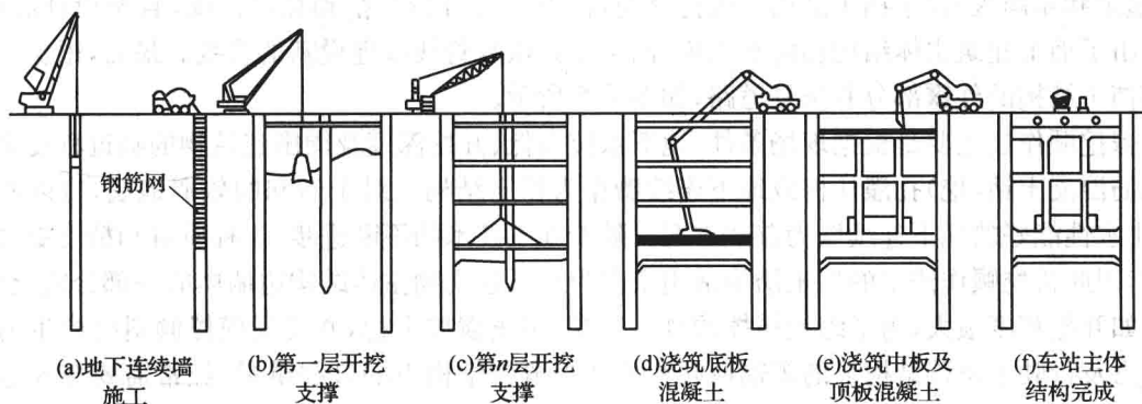
图 1.1 明挖法车站施工工序
