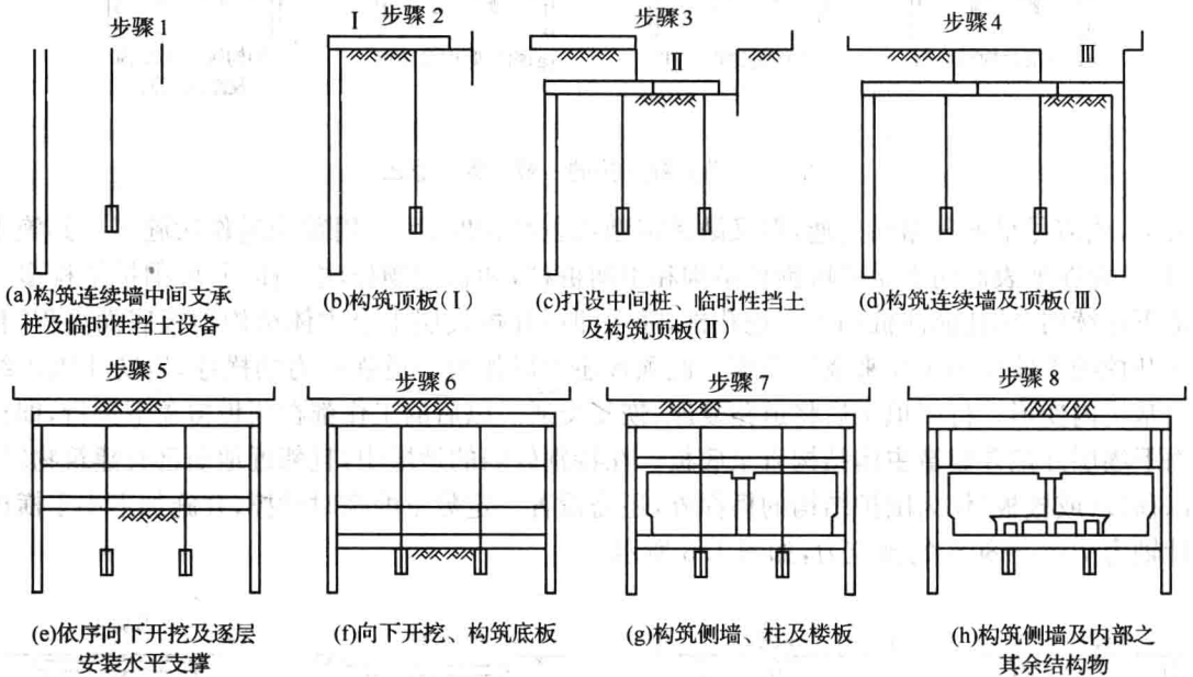
图 1.4 盖挖半逆作法施工步骤
