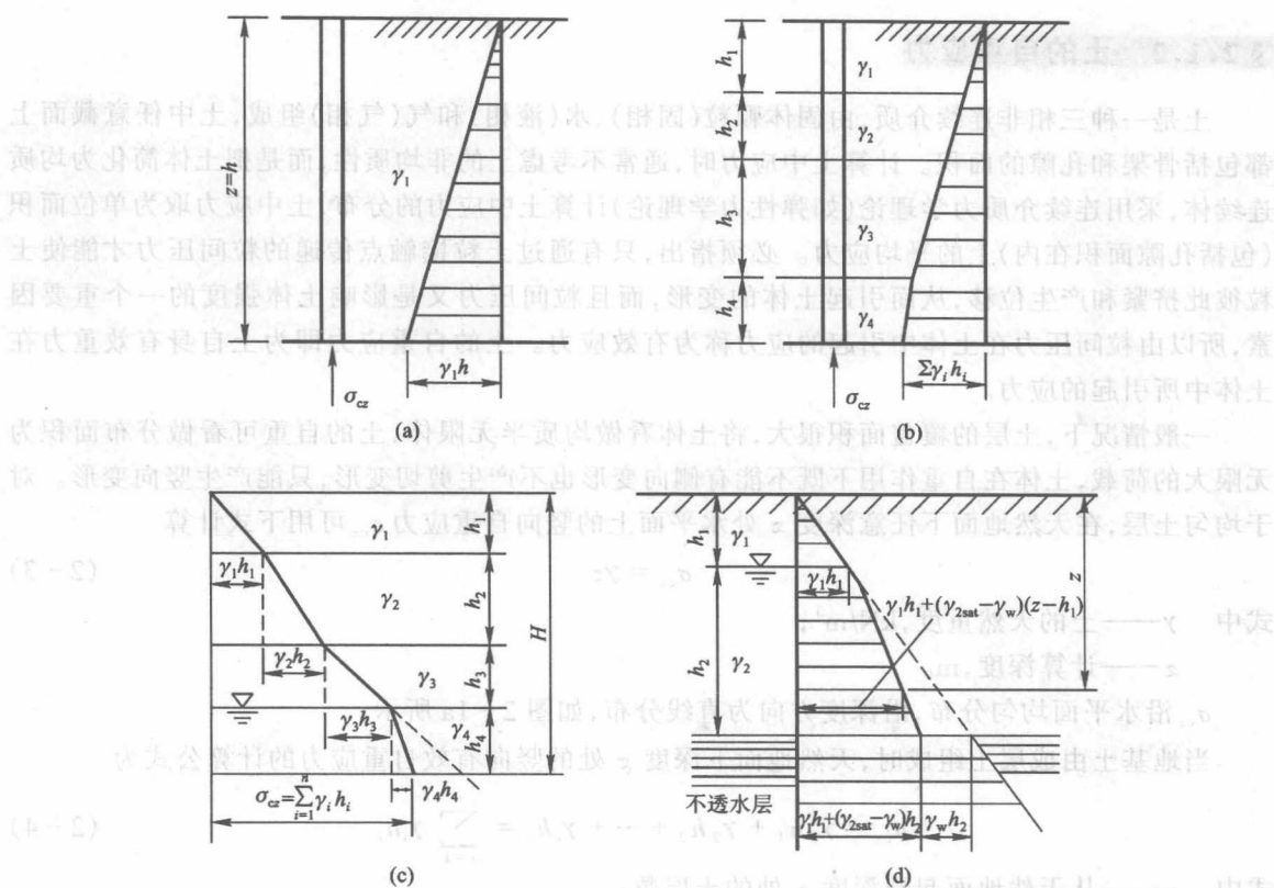
图 2-1 土的自重应力分布
