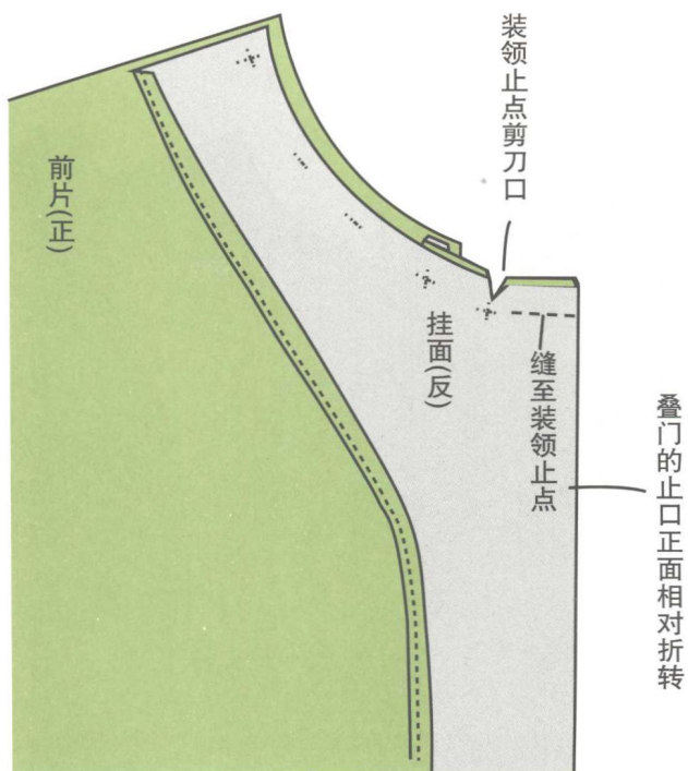
3-5 装领止点剪刀口。
