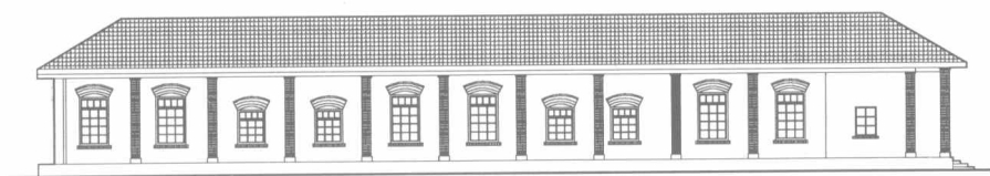
南立面图
