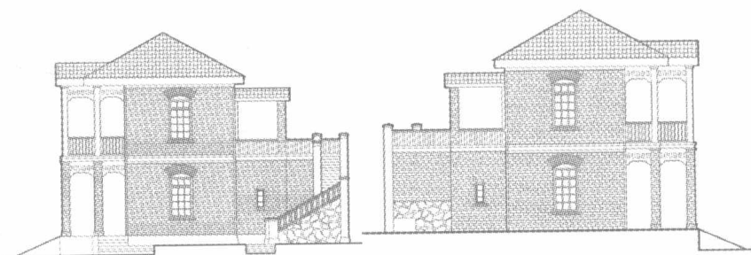
南立面图
