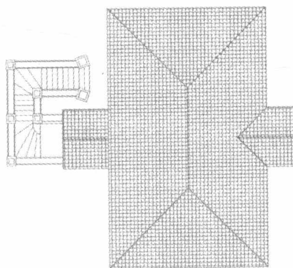
屋顶平面图
