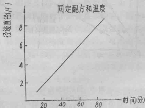
图 4 径迹直径与蚀刻时间的关系
