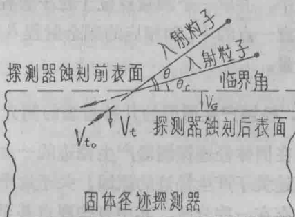
图 9 \theta_c , V_t 和 V_G 示意图
