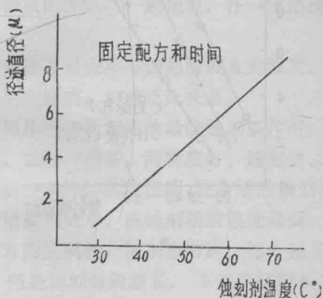
图 3 径迹直径与蚀刻温度的关系
