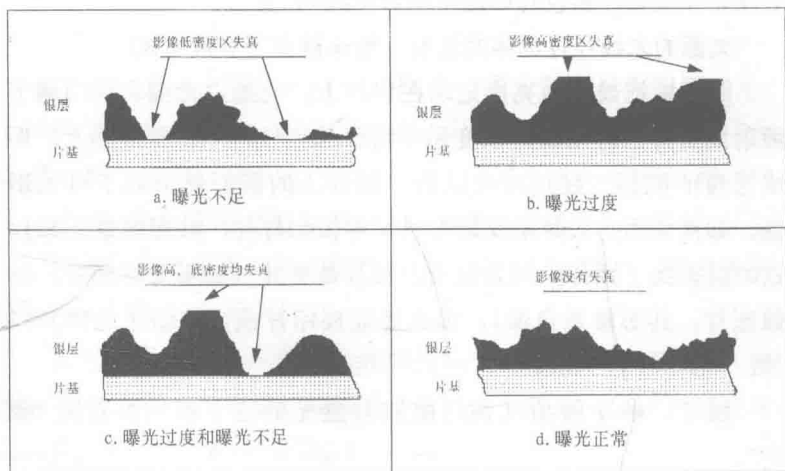
图 1-2 胶片不同曝光情况示意
