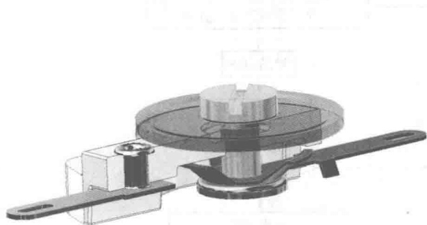
图 1-2 微调瓷介质电容器的三维装配立体图(剖开)
