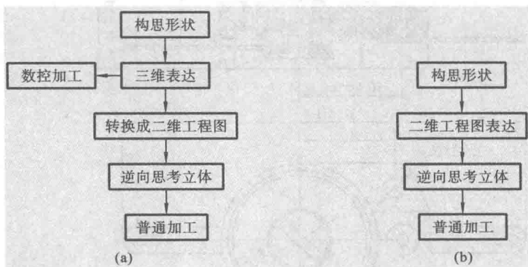
图 1-5 产品的两种设计方式
