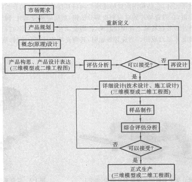
图 1-1 产品的设计过程
