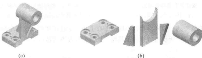
图 2-3 杠杆开关支座及其分解图
