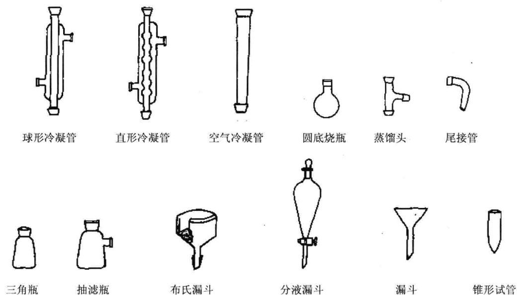
图 1-3 微型实验仪器
