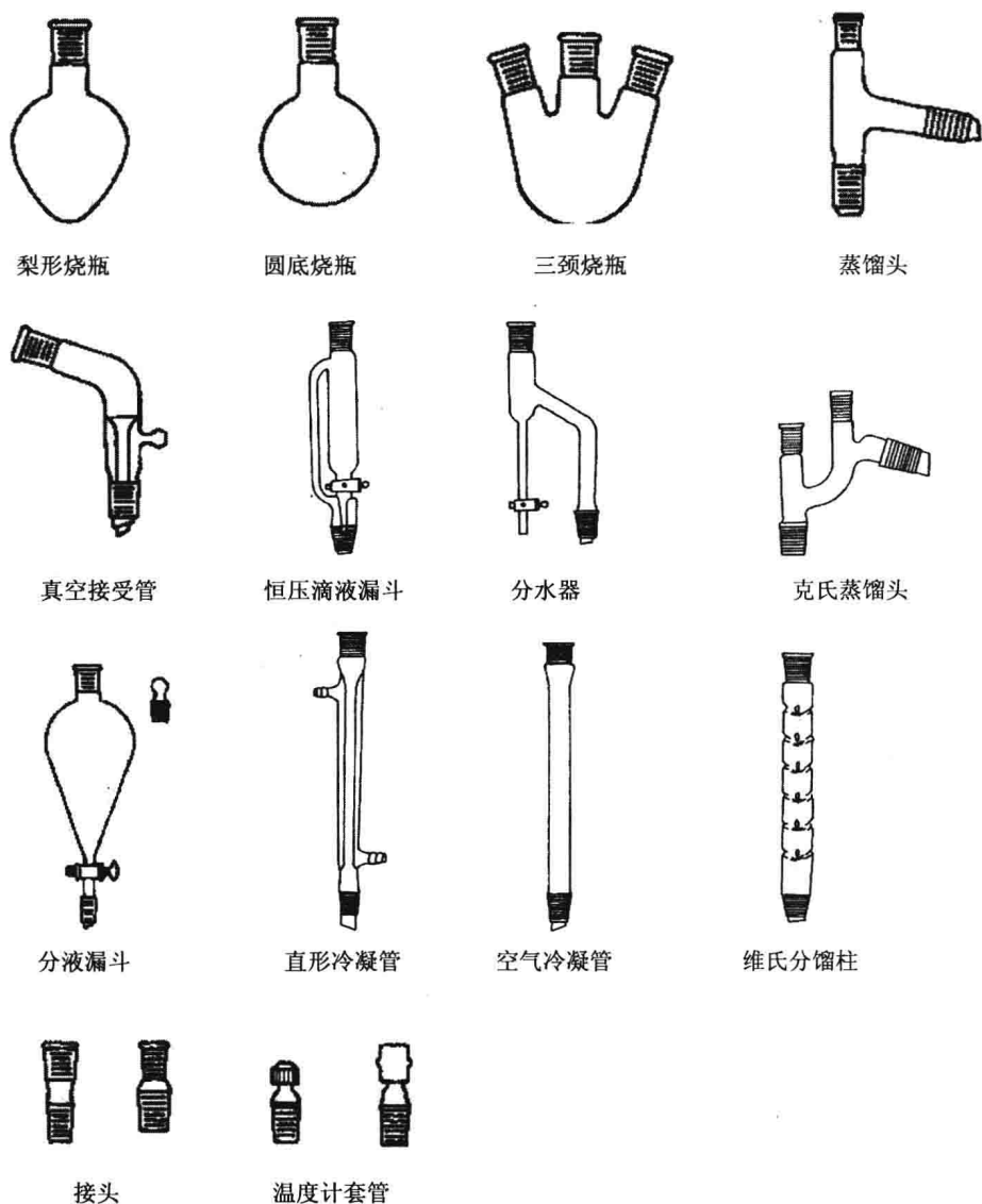
图 1-2 标准磨口仪器
