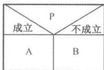
图 1-6 选择结构
