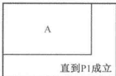
图 1-8 直到型循环
