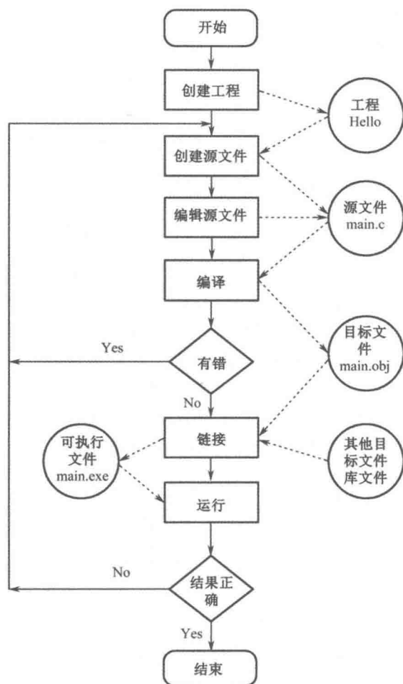
图 1-1 运行 C 程序的步骤和方法
