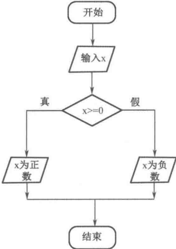
图 1-4 例 1-3 流程图
