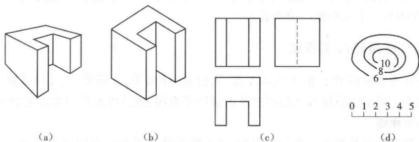
图 1-9 工程上常用的四种投影图
