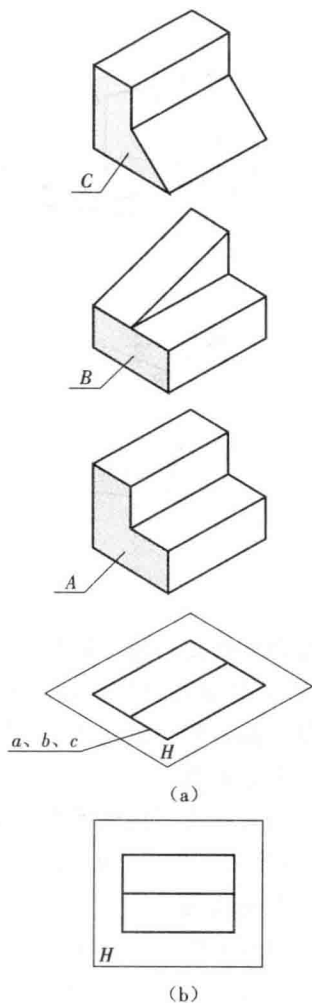
图 1-4 形体的单面投影
