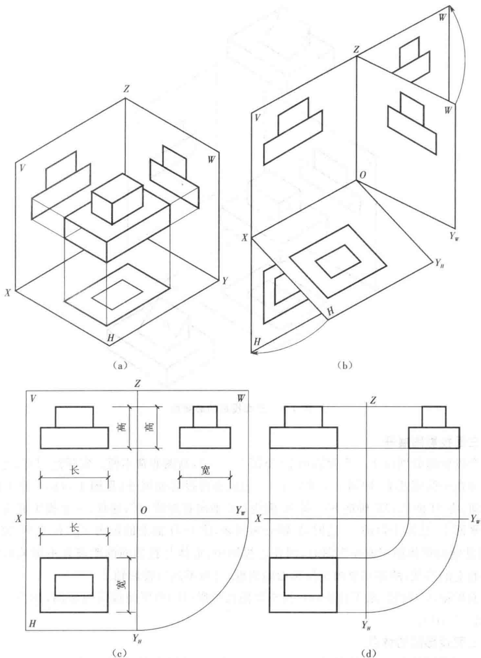
图 1-7 三投影面体系和三面投影图
