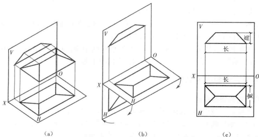
图 1-5 四坡顶屋面的两面投影
