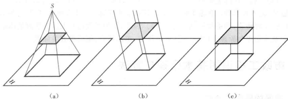
图 1-2 投影法的分类
