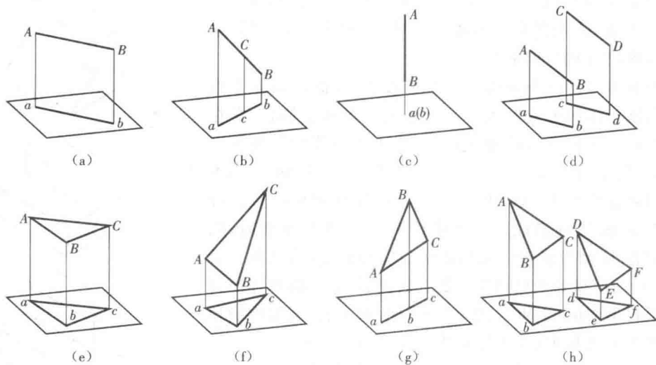
图 1-3 正投影的基本性质
