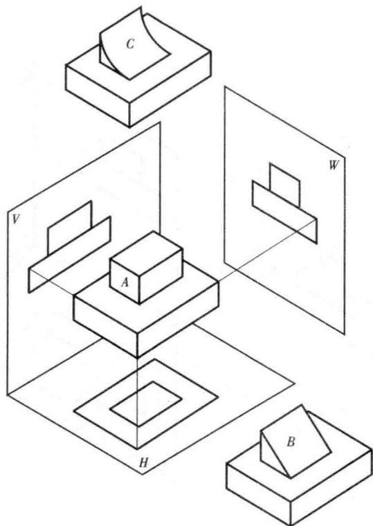
图 1-6 三面投影的必要性
