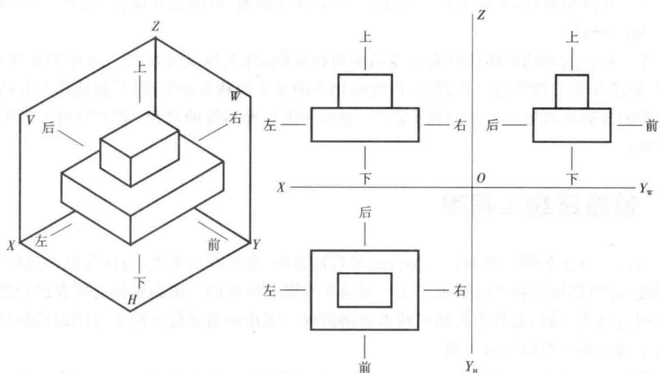
图 1-8 投影图上形体方向的反映
