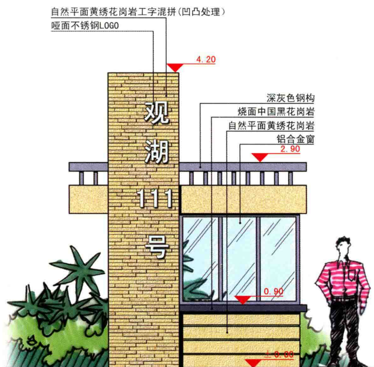
西入口岗亭正立面图
