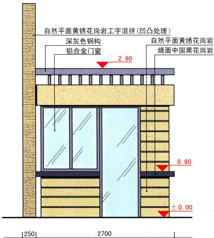
西入口岗亭侧立面图
