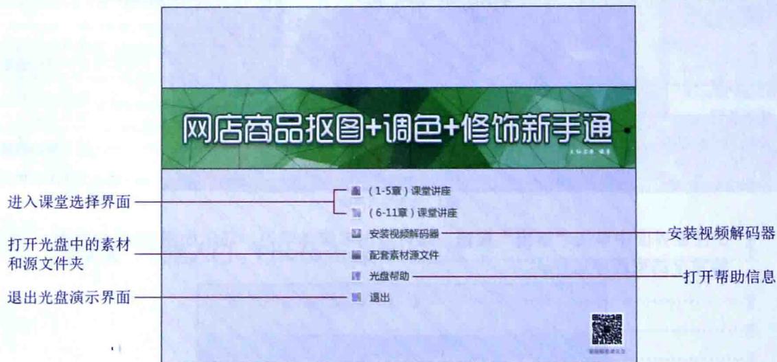
图1 主界面
