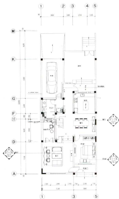
一层平面布置图
