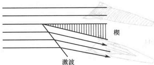
图 1.2.4 流经二维的超声速流动
