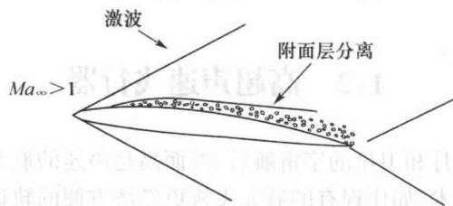
图 1.1.2 激波引起阻力的示意图
