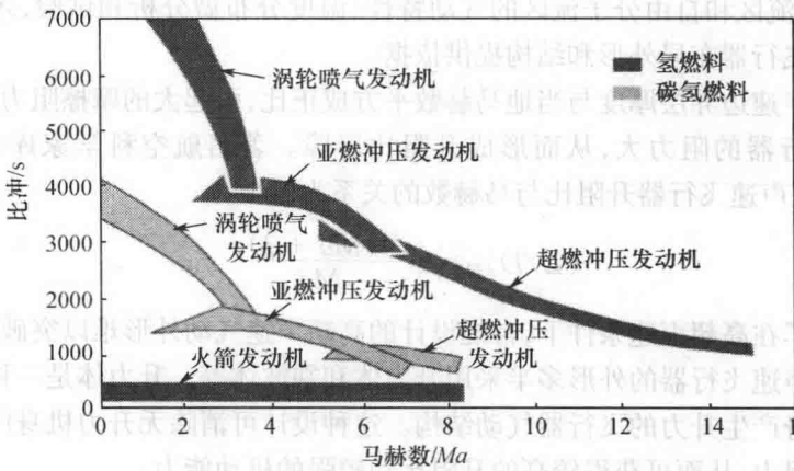
图 1.2.3 超声速发动机发展趋势
