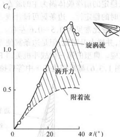
图 1.3.2 细长机翼的涡升力
