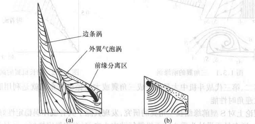
图 1.3.4 边条翼对主翼流态的有利影响 (a) 边条翼; (b) 基本翼。
