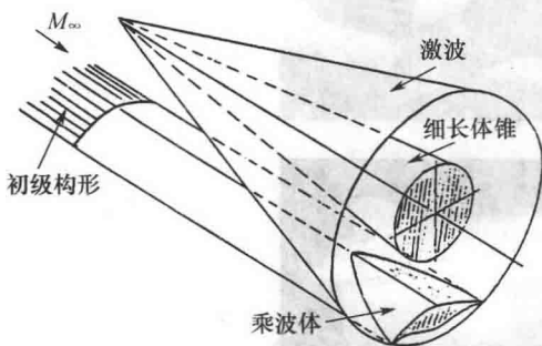
图 1.2.6 一种曲面型乘波机翼方案
