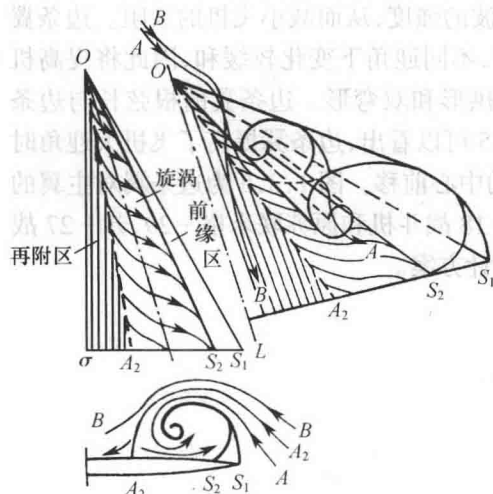
图 1.3.1 三角翼的前缘涡
