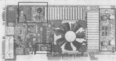
(图2)采用公板PCB设计的GeForce3 Ti500
