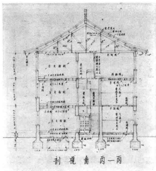
剖面圖
