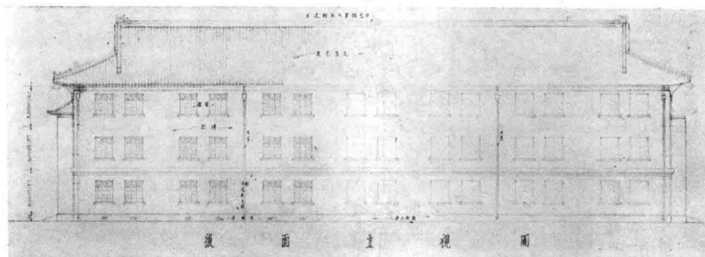
後面立視圖
