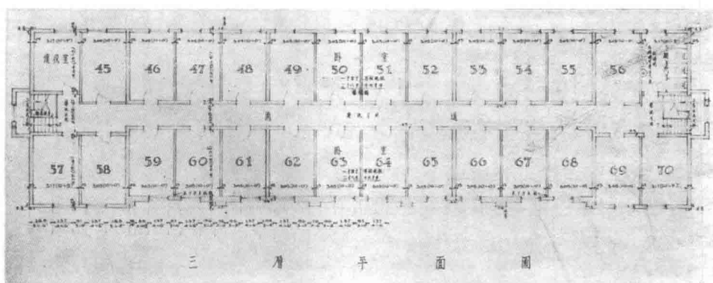
男生宿舍平面圖
