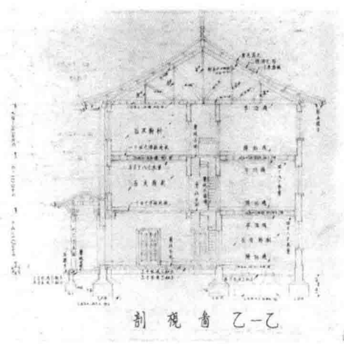
剖面圖
