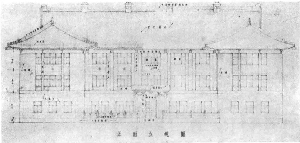
正面立視圖
