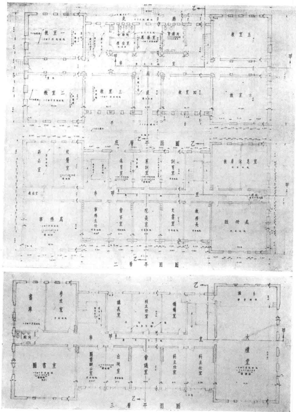
辦公廳及教室平面圖
