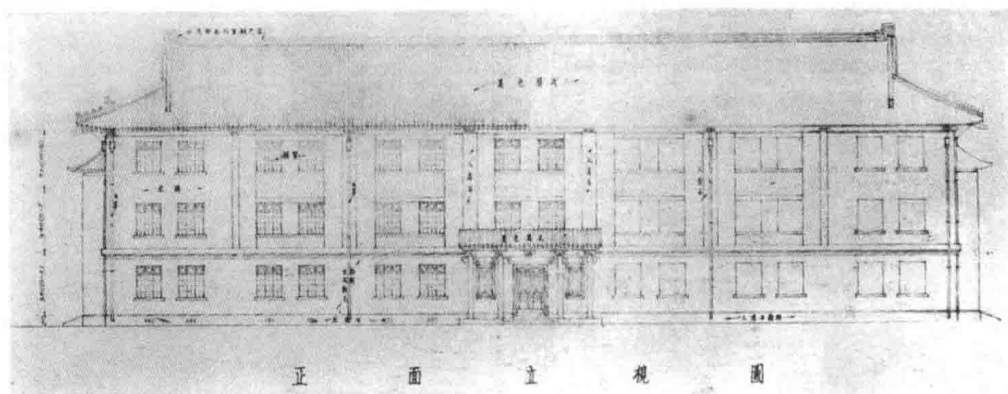
正面立視圖
