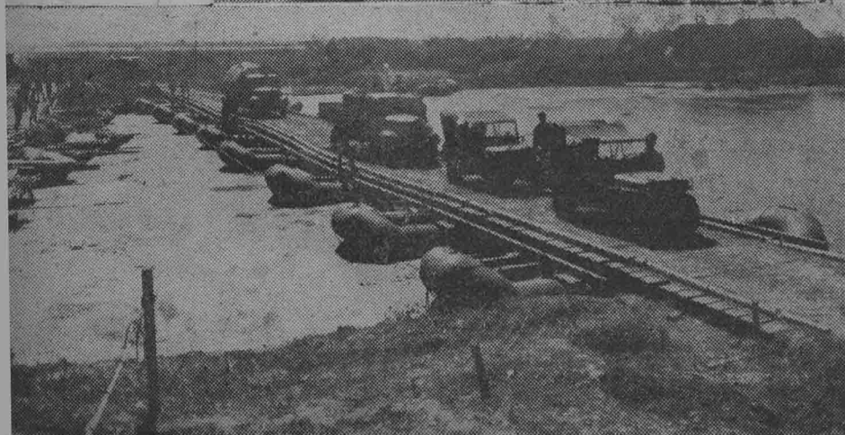
橋基穩固通過大批 重車輛 (南通陸軍工兵第二 團攝) → ←
