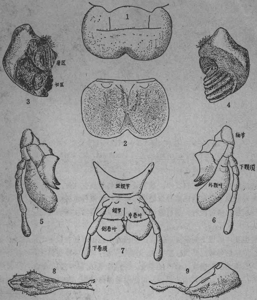
图 1—5 蝗虫的口器
