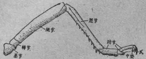
图 I—14 蝗虫的前足
