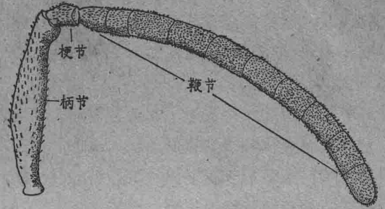
图 I—3 蜜蜂的触角
