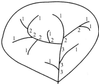
图 1-1 流域和水系 1~3—河流的级别
