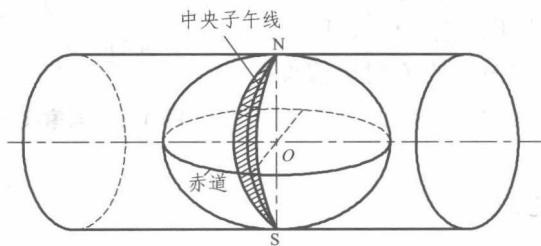
图 1.5 高斯投影
