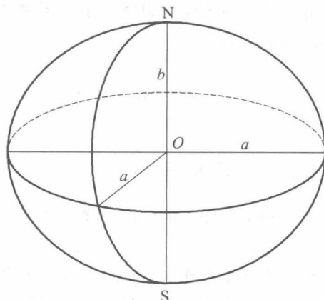
图 1.2 旋转椭球体
