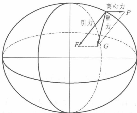
图 1.1 引力、离心力和重力
