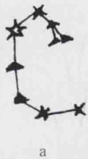
8 玉片九孔与星宿对应关系 a 星宿星象示意 b 玉片九孔示意 c 玉片九孔弯曲示意 (引自王育成《含山玉龟玉片补考》)
