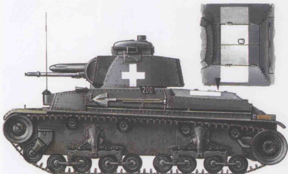
■ 35 (t) 型坦克。
