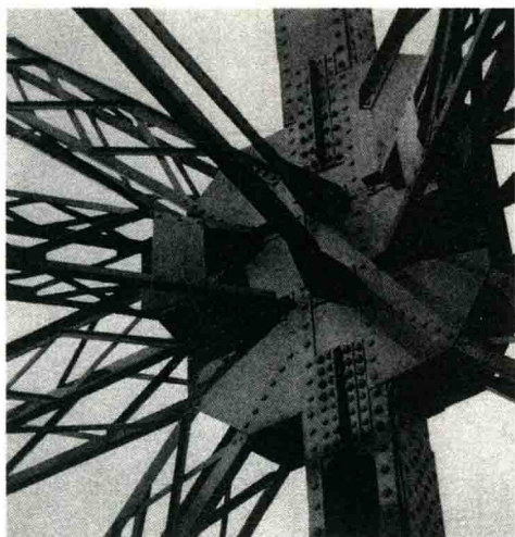
埃菲尔铁塔的结点组成，巴黎，1889年
