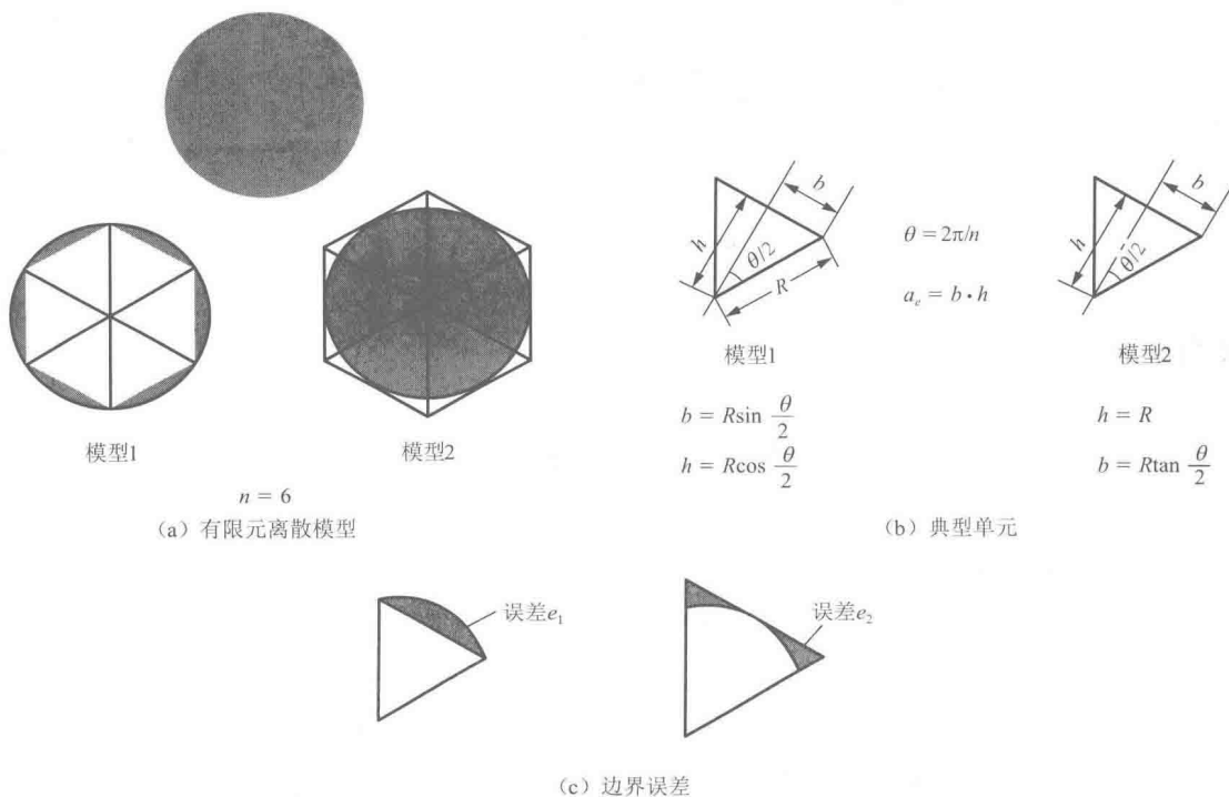
图 1-2 圆的有限元模型
