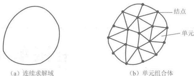
图 1-1 有限单元法图解
