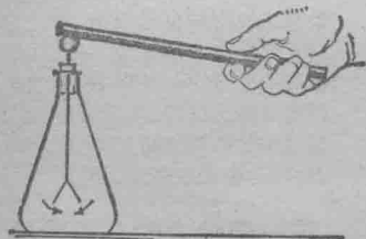
图 18.5 用一根石墨棒接触带电验电器小球时,两片金箔下落,说明人体和石墨都是导体。
