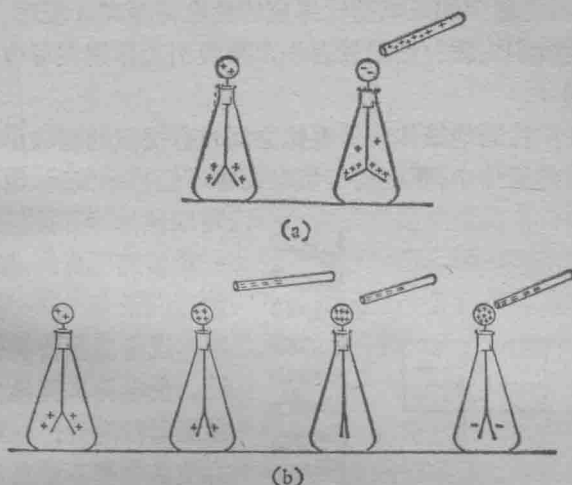
图 18.8 用验电器探测电荷，确定其正负。在 (a) 中把正电荷移近一个带正电的验电器，两片金箔的张角加大。在 (b) 的一系列图中，把负电荷逐渐移近带正电的验电器小球，越来越多的负电荷被排斥到两片金箔上，因而金箔逐渐下落。最后，如果大量负电荷离得很近，可能把如此多的负电荷排斥到金箔上，致使两片金箔带上净负电荷，其张角又会加大。
