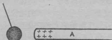
图 18.9 对中性导体的吸引作用。当一个中性导体靠近一个带正电的物体时，导体中负电荷被吸引至靠近正电荷的一端，而正电荷留在导体远端。由于感生负电荷距离带正电的物体较近，所以有净吸引力存在。
