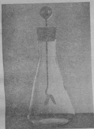
图 18.3 金箔验电器。两片金箔由于带电而张开。
