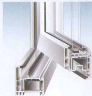
欧洲之翼70MD平开门窗系统
