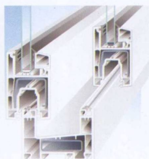
坚固先锋78推拉门系统
