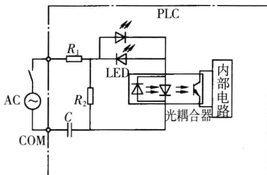
(c) 交流输入电路
