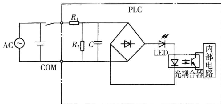
(b) 交流 / 直流输入电路
