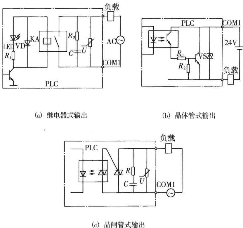
图 1-3 开关量输出接口电路
