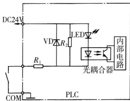
光耦合
