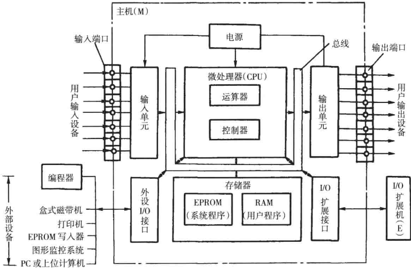
图 1-1 PLC 硬件结构简化框图
