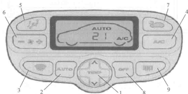
1—温度调节按钮；2—自动空调启动钮；3—空气流量控制；4—空调启动开关； 5—车内空气分配控制；6—空气流量控制；7—进气控制；8—空调关闭开关； 9—后风窗除霜控制
