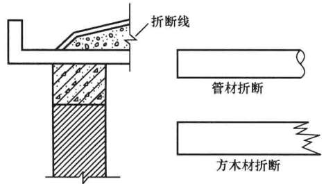
图 1-10 折断线表示方法
