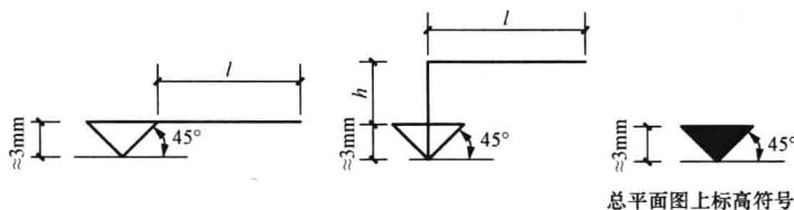
图 1-13 标高绘法
