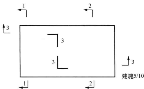
图1-5 剖切标志法
