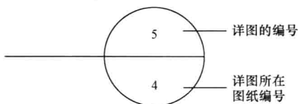
图 1-18 详图索引在其他图
