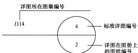
图 1-19 标准图索引
