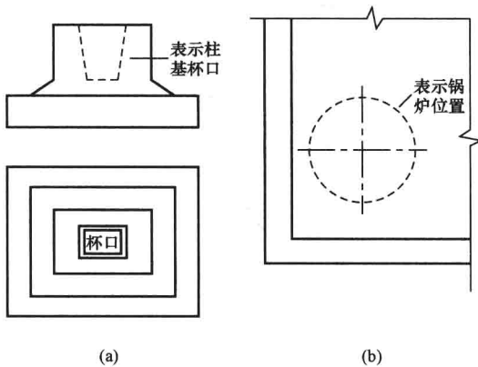
图 1-11 虚线表示方法
