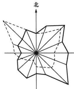
图 1-16 风玫瑰
