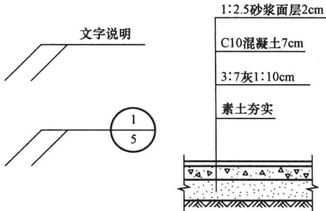
图 1-9 引出线表示方法
