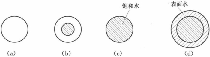
图 1.3 材料的含水状态 (a) 干燥状态；(b) 气干状态；(c) 饱和面干状态；(d) 湿润状态
