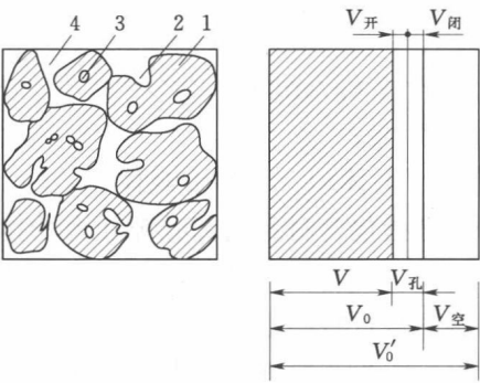
图 1.2 散粒材料体积构成示意图 1—颗粒中固体物质；2—颗粒的连通孔隙；3—颗粒的封闭空隙；4—颗粒间的空隙
