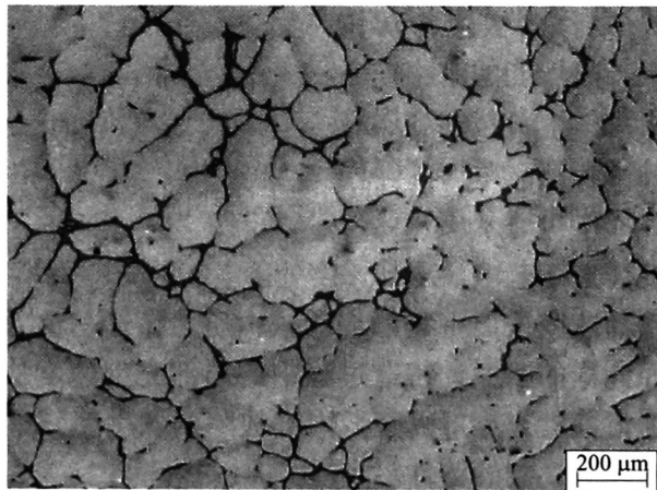
图 1.4 AlCu 4 合金材质砂型铸件的显微结构
