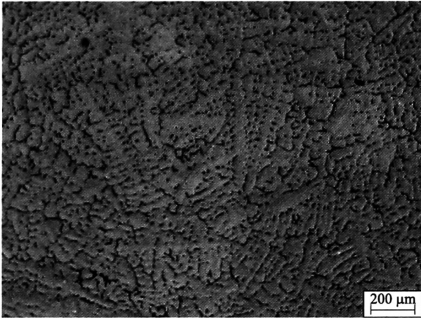
图 1.5 AlCu 4 合金材质硬模铸件的显微结构
