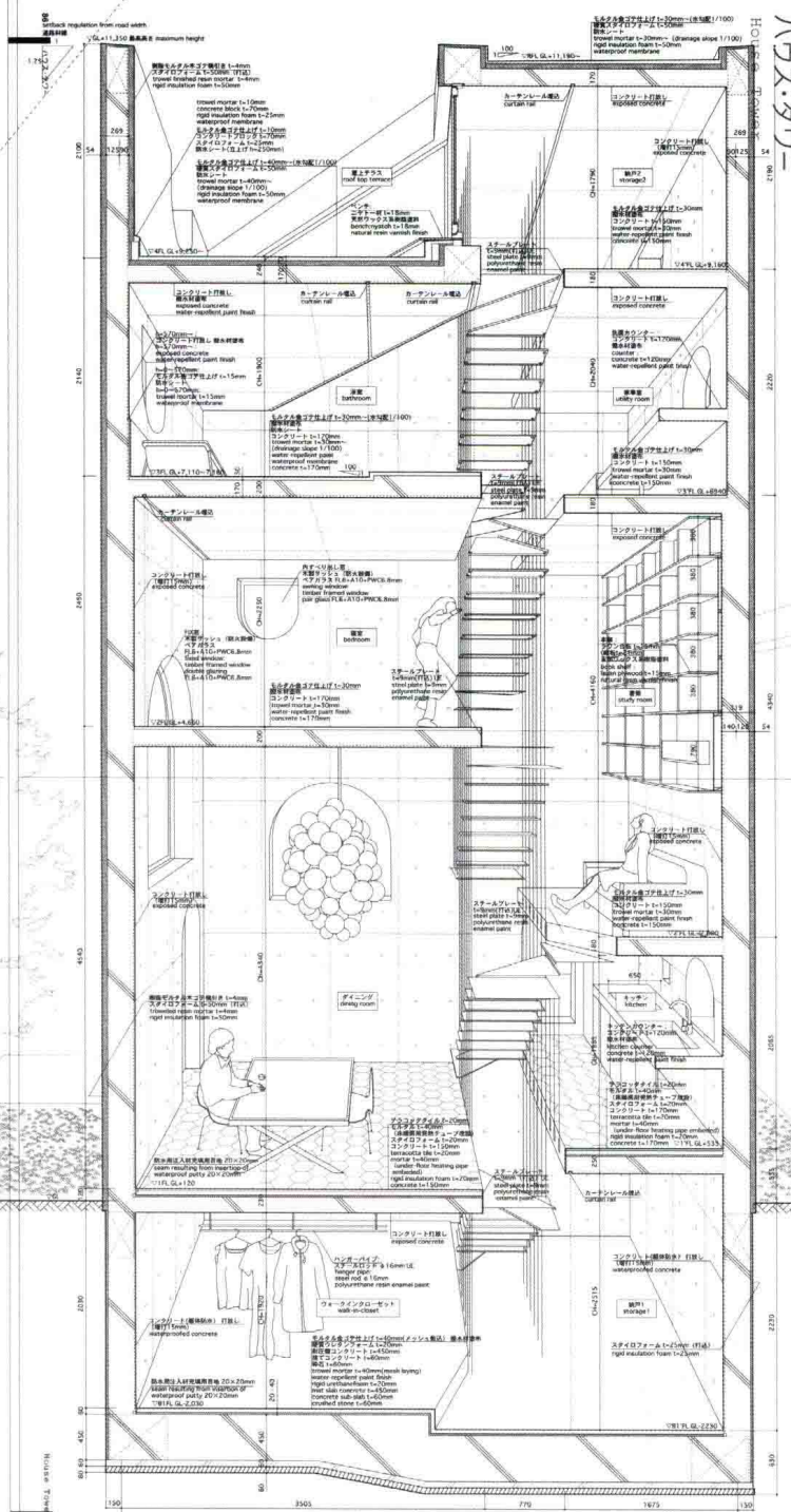
断面詳細バース / vertical section perspective S:1/30
