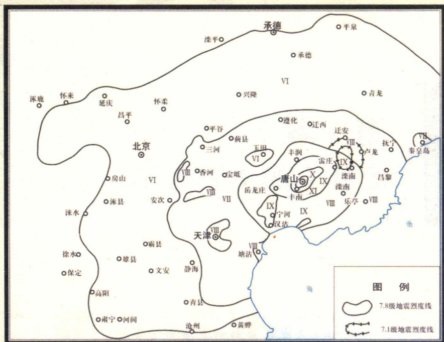
唐山地震区烈度分布图
