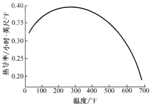
图 1.7 轻水(液体)的热导率 ③
