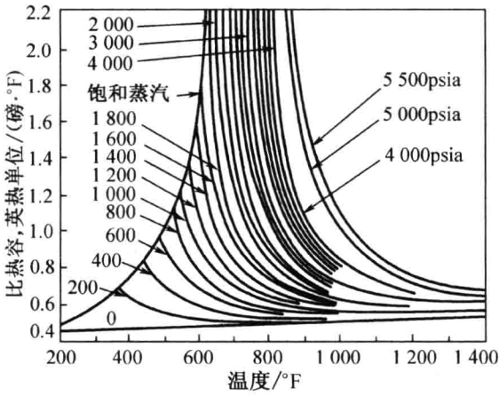
图 1.10 轻水蒸气的比热
