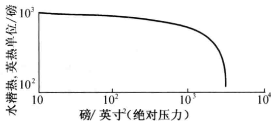
图 1.8 轻水的蒸发潜热
