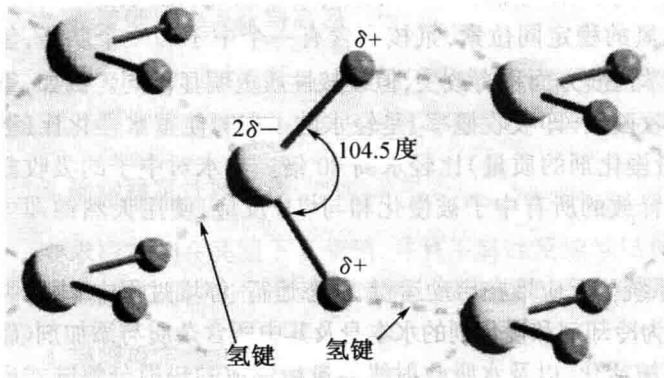
图 1.2 液态和固态水中荷正电的氢原子和荷负电的氧原子之间形成的氢键
