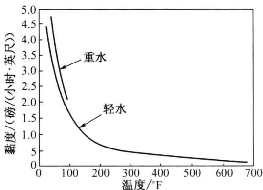
图 1.6 轻水和重水的黏度 ②
