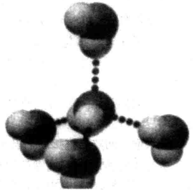
图 1.3 水分子间的氢键
