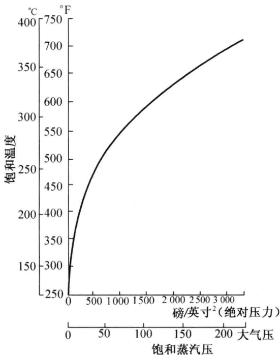
图 1.9 轻水的蒸汽压
