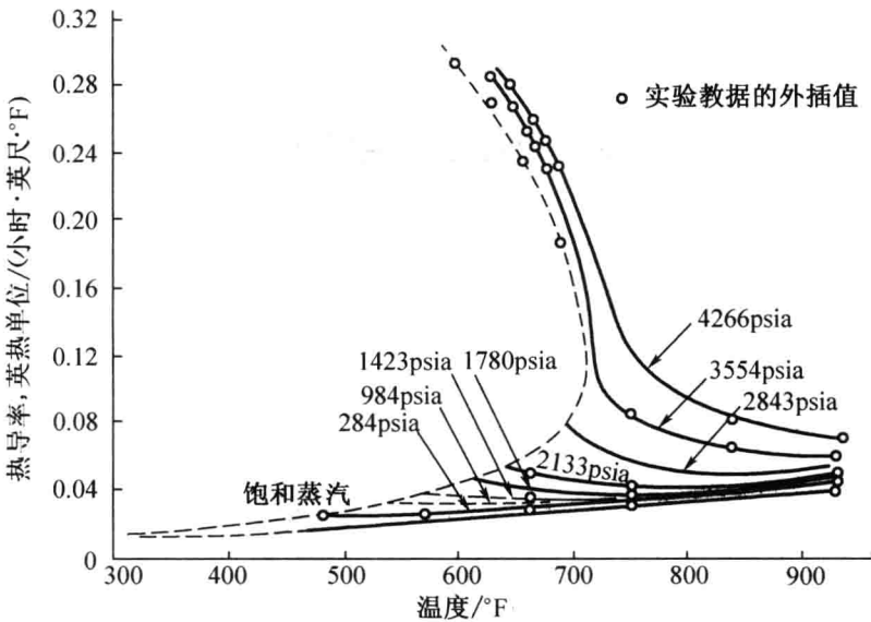
图 1.12 轻水蒸气的热导率
