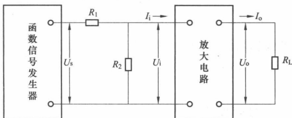
图 1-3 分压法测量放大倍数
