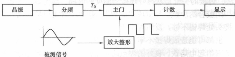
图 1-1 频率计工作原理框图
