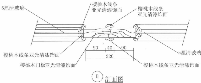
▲003-豪华装饰门大样(三)
