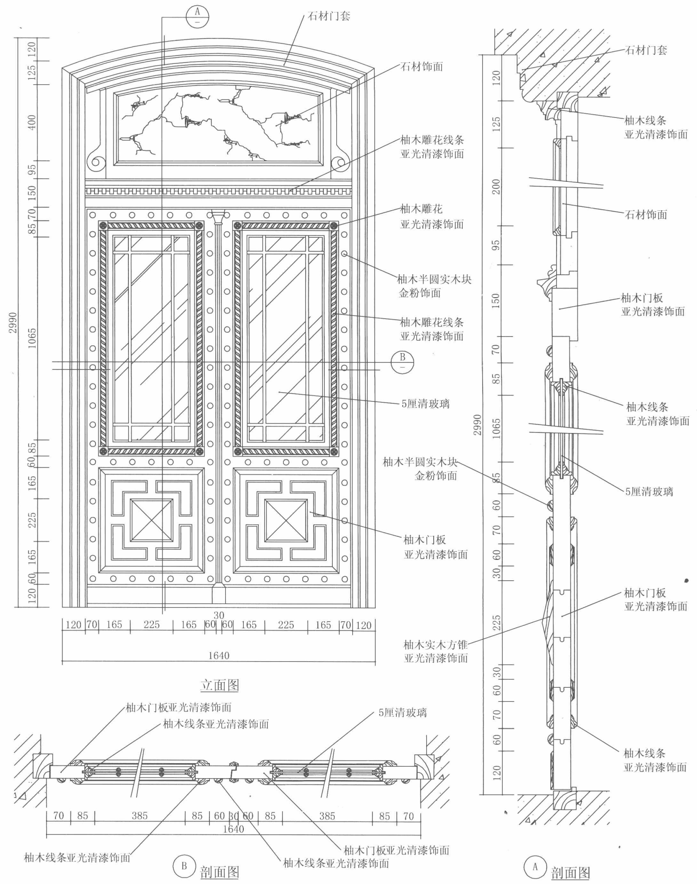
▲001-豪华装饰门大样 (一)
