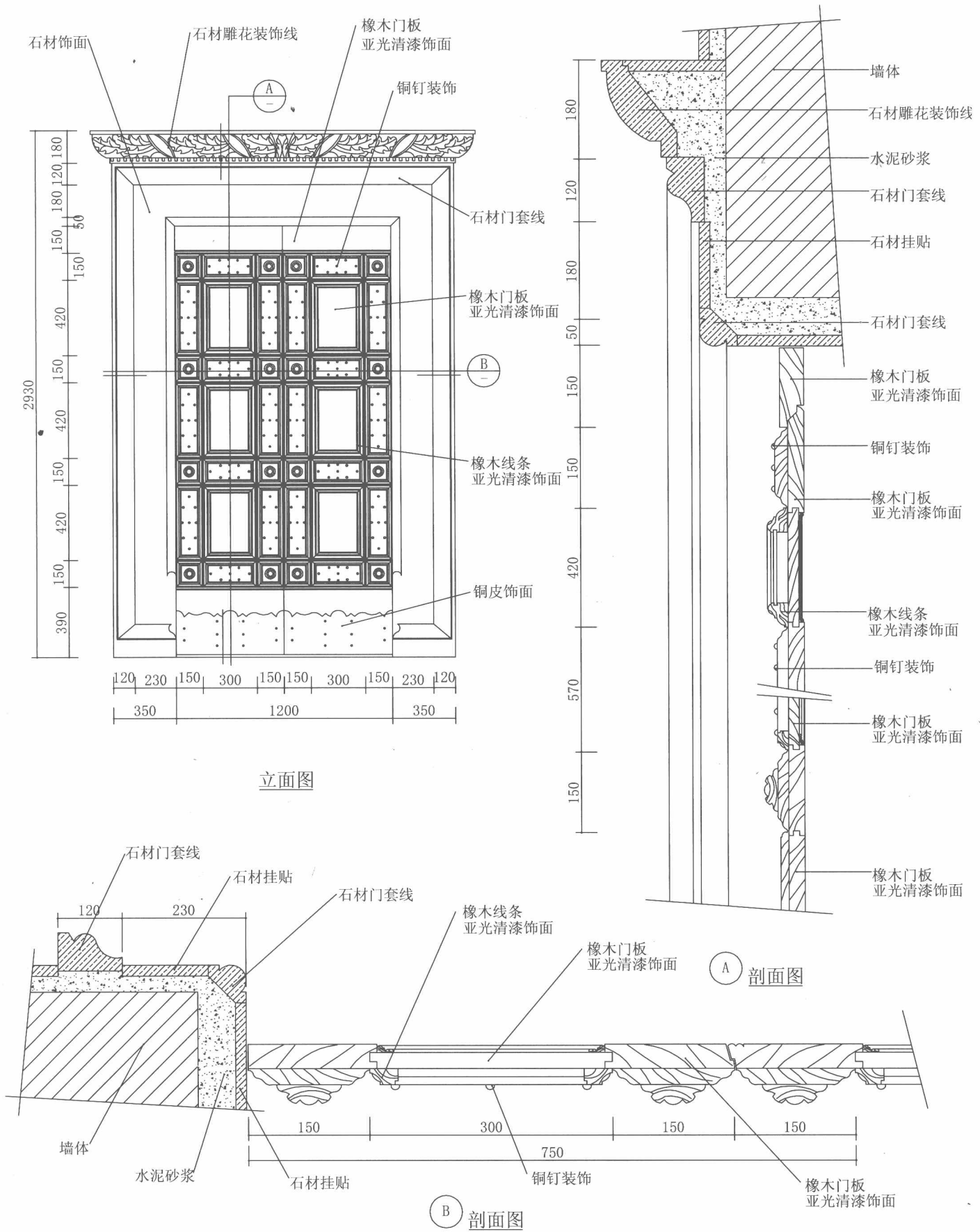
▲002-豪华装饰门大样(二)
