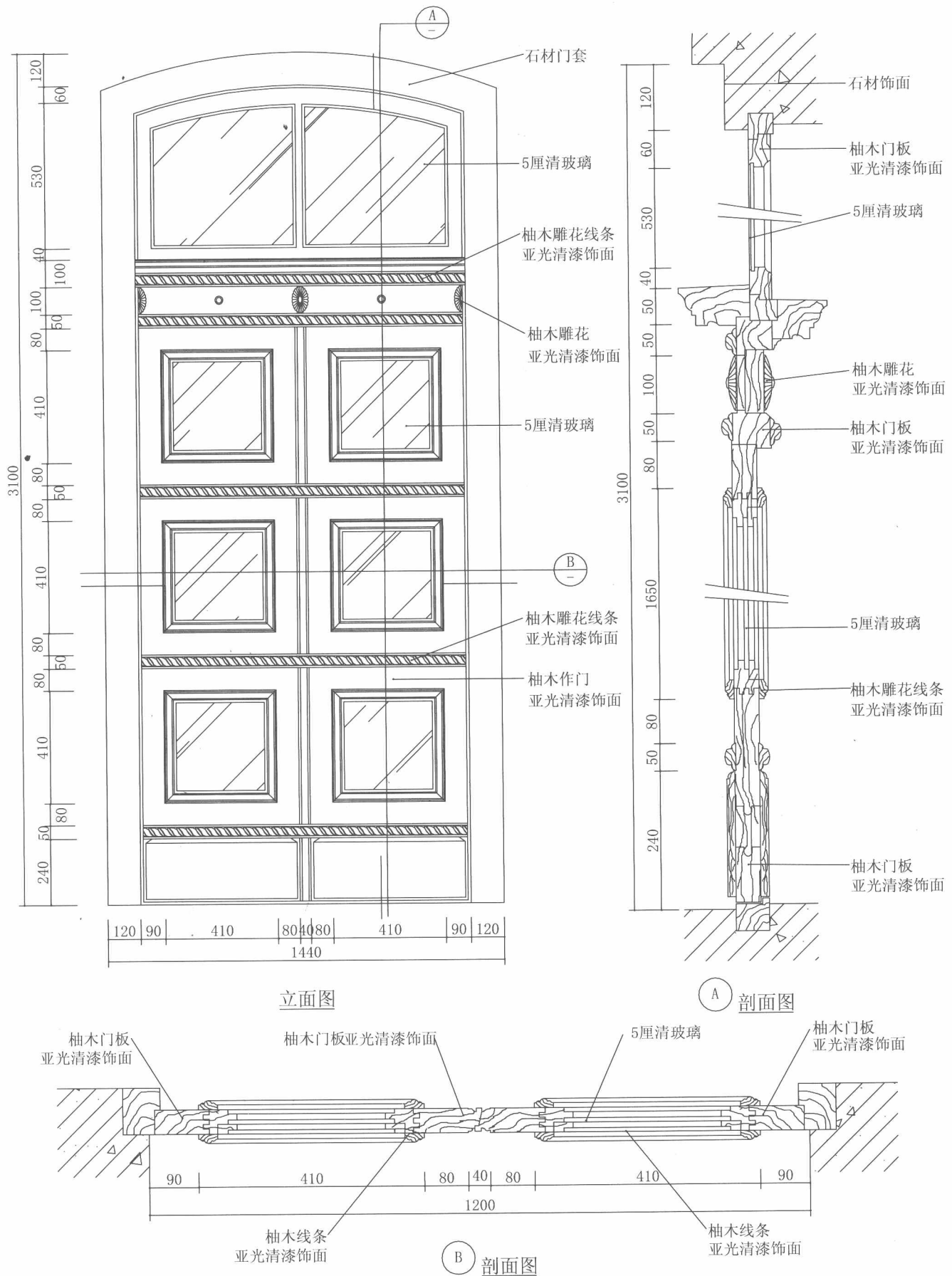
▲004-豪华装饰门大样 (四)
