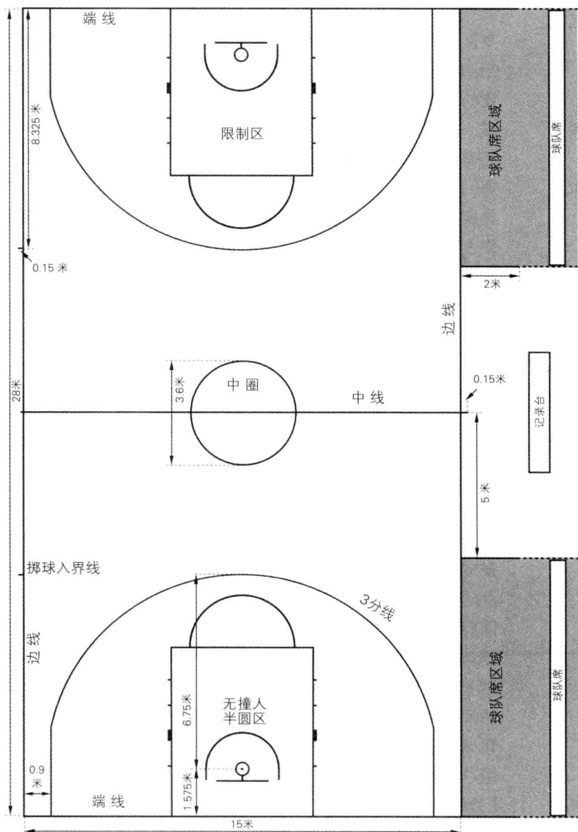
图1 比赛场地的全部尺寸
