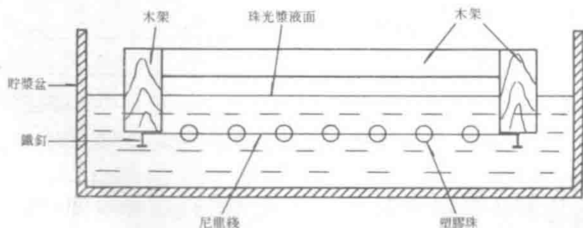
圖 4 浸塗塑膠珠時情況
